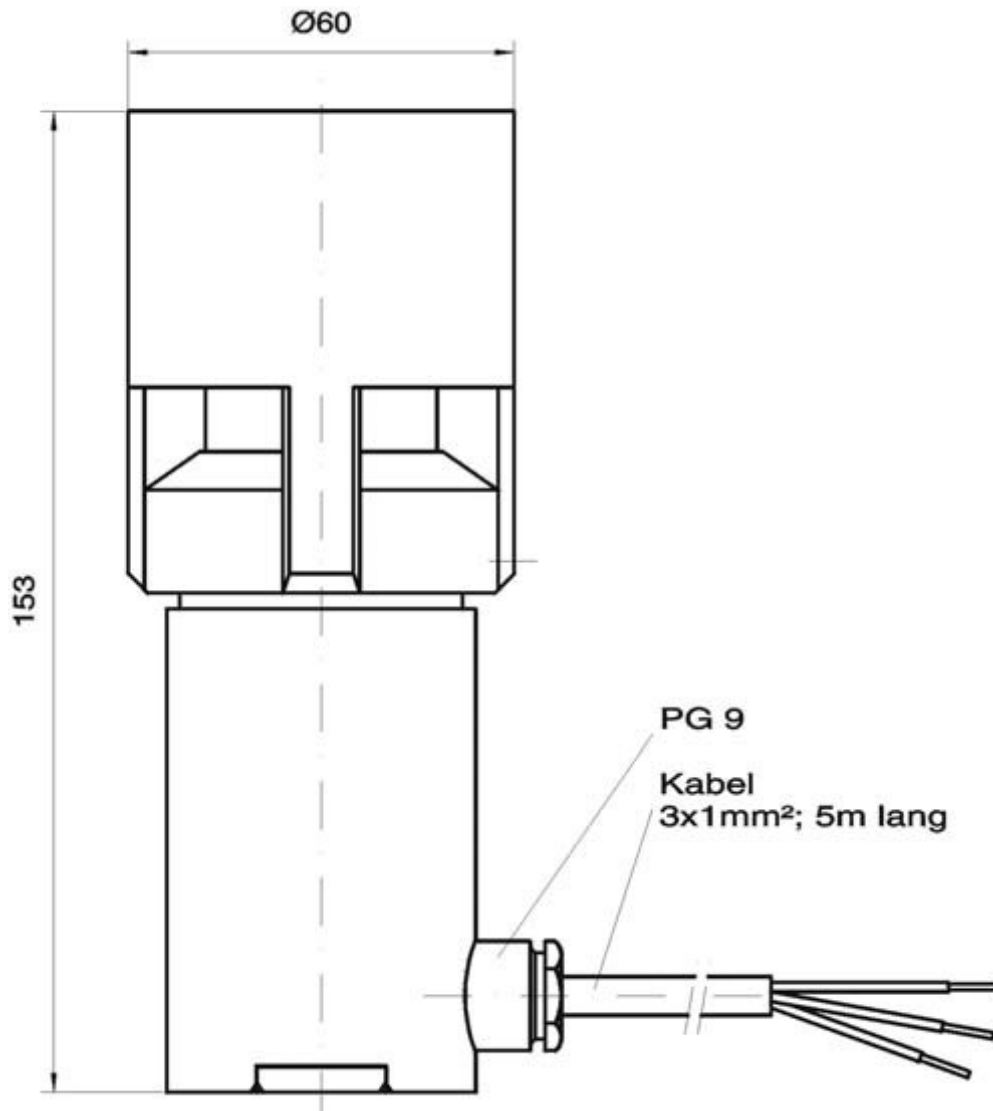
Abbildung 1: Abmessungen
