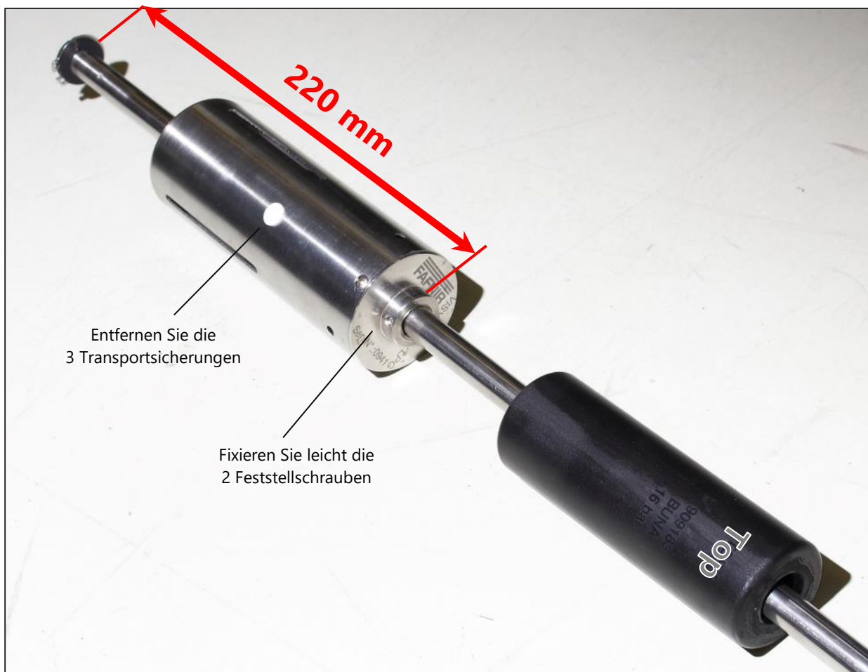
Abbildung 5: Zubehör Montage (maximale Konfiguration)
