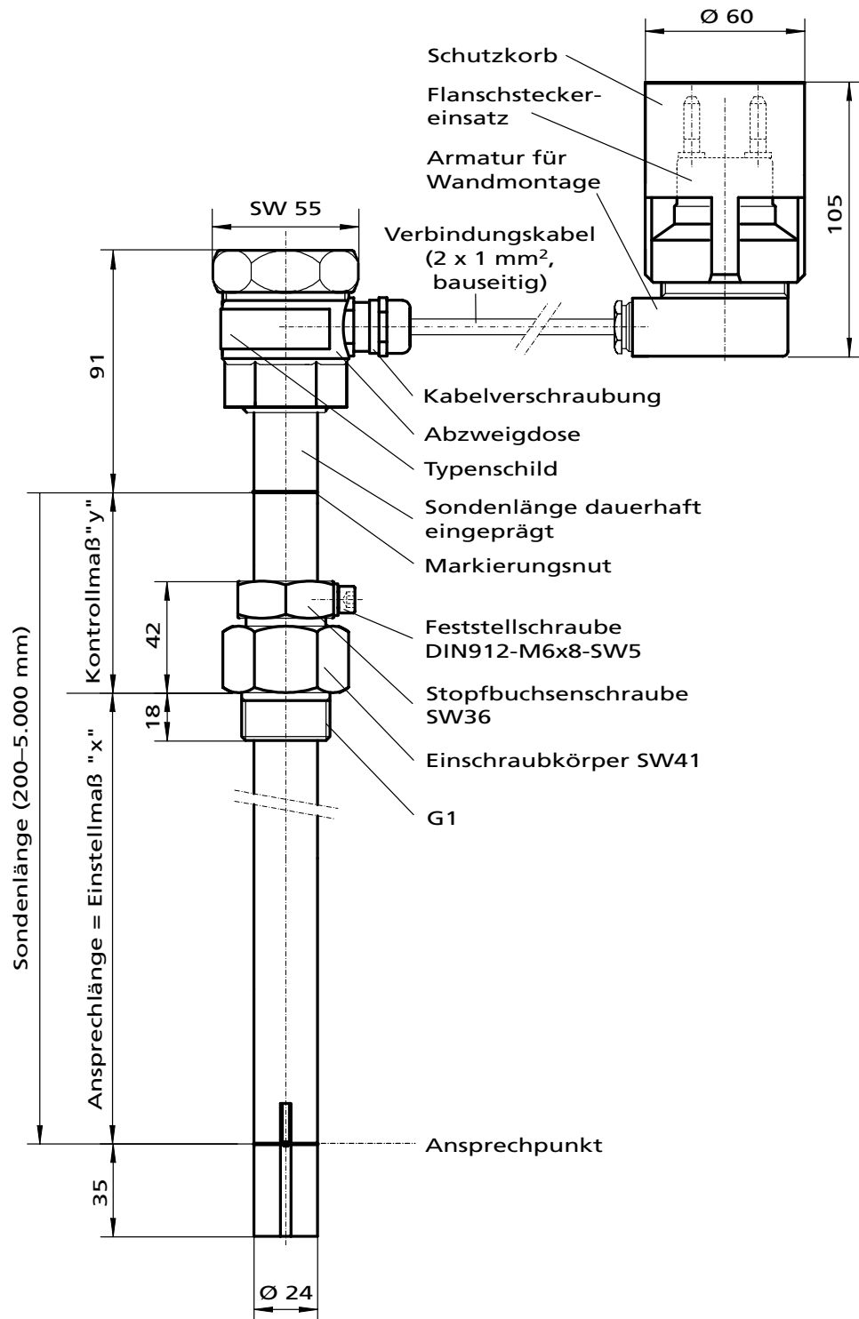
Abb 2b: Grenzwertgeber Typ FAFNIR 83 UV mit Wandarmatur
