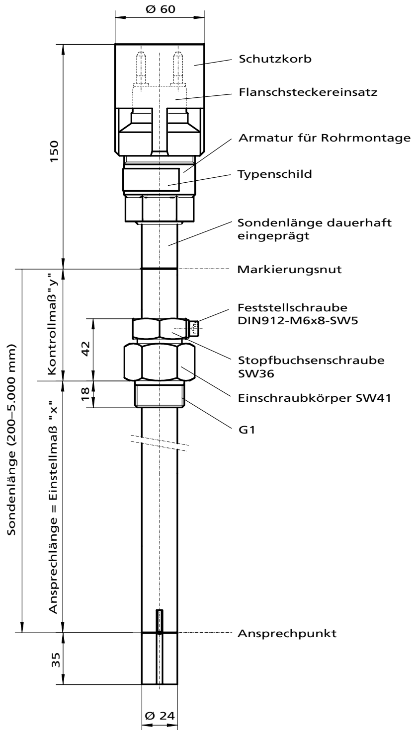
Abb. 2a: Grenzwertgeber Typ FAFNIR 83 UV mit Rohrarmatur
