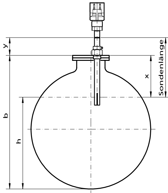
Abb. 1a: Tanks nach DIN 6608, 6616, 6617, 6624 und TGL 5315
