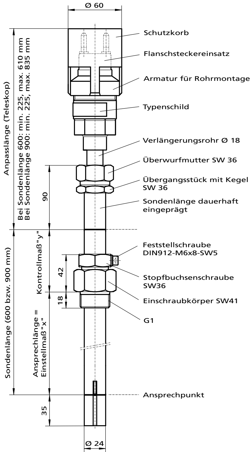
Abb. 3: Grenzwertgeber Typ FAFNIR 84 UVT mit Rohrarmatur
